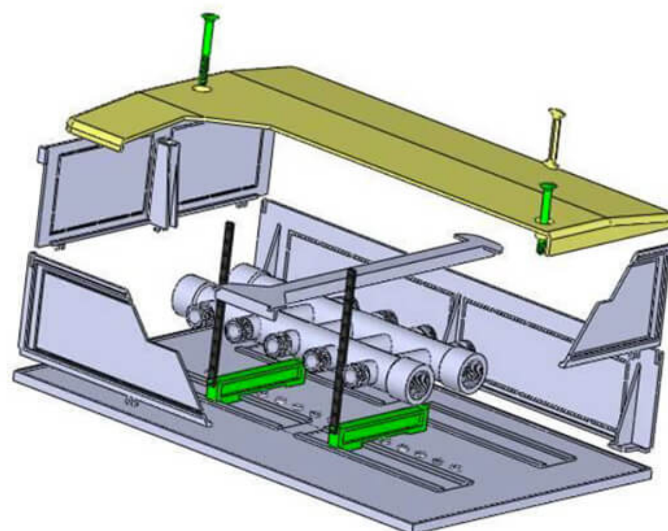
COLLETTORE COMPLANARE
